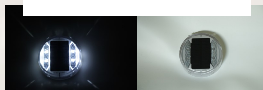
ILSE-308 : dia 110 x 35 mm
